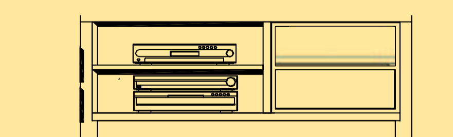
Lowboard 7024-01 2 Fächer, 2 Schübe B 138 x T 50 x H 52 cm
