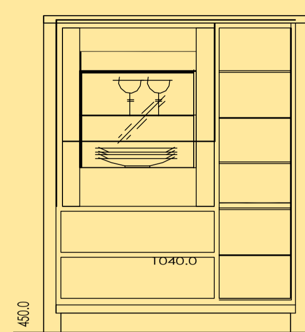
Kommode 7060-01 2 Türen, 2 Schübe B 104 x T 45 x H 124 cm
